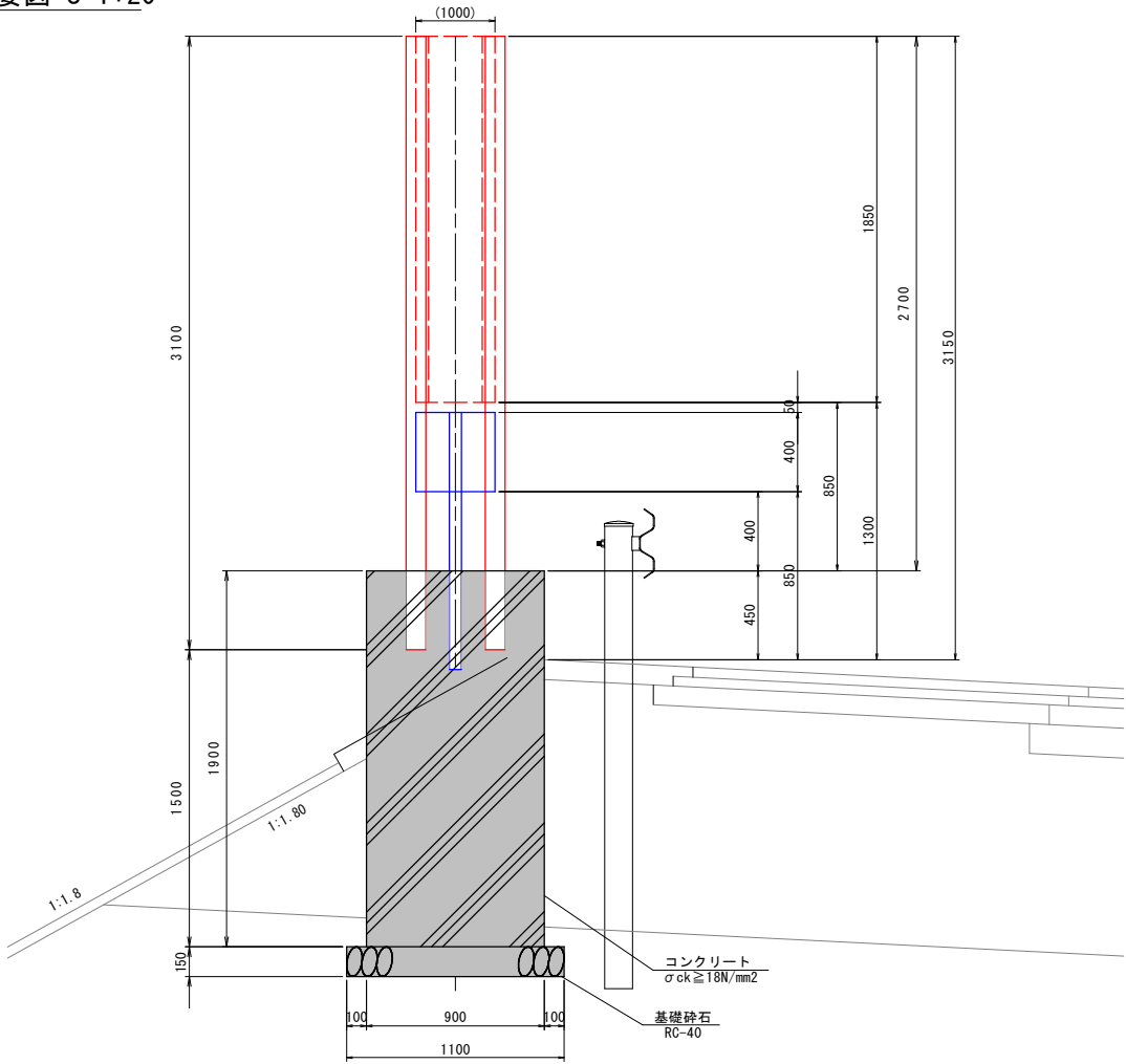
左法肩部 姿図 S=1:20
